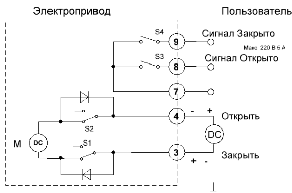
Рис. 2в Принципиальная электрическая схема подключения электропривода САТУРН ЭП-Ч к сети 24 В (Исп. 24VDS)
