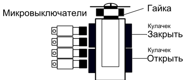
Рис. 8а Настройка конечных выключателей приводов САТУРН ЭП-Ч 003-015
