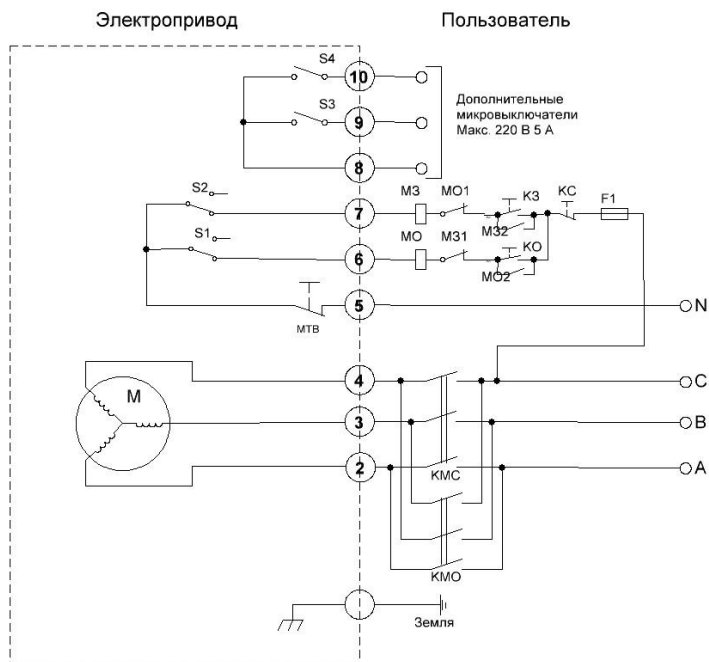
Рис. 26 Принципиальная электрическая схема подключения электропривода САТУРН ЭП-Ч к сети 380 В, 50 Гц (Исп. К3)
