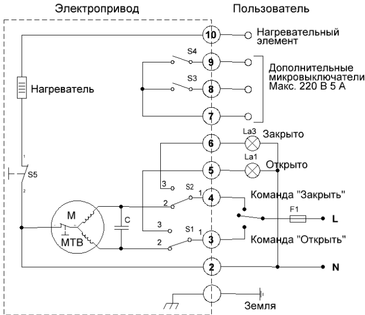
Рис. 2а Принципиальная электрическая схема подключения электропривода САТУРН ЭП-Ч к сети 220 В, 50 Гц (Исп. S01- стандартное, нагревательный элемент – опция, в ЭП-Ч 003 установка не возможна)
