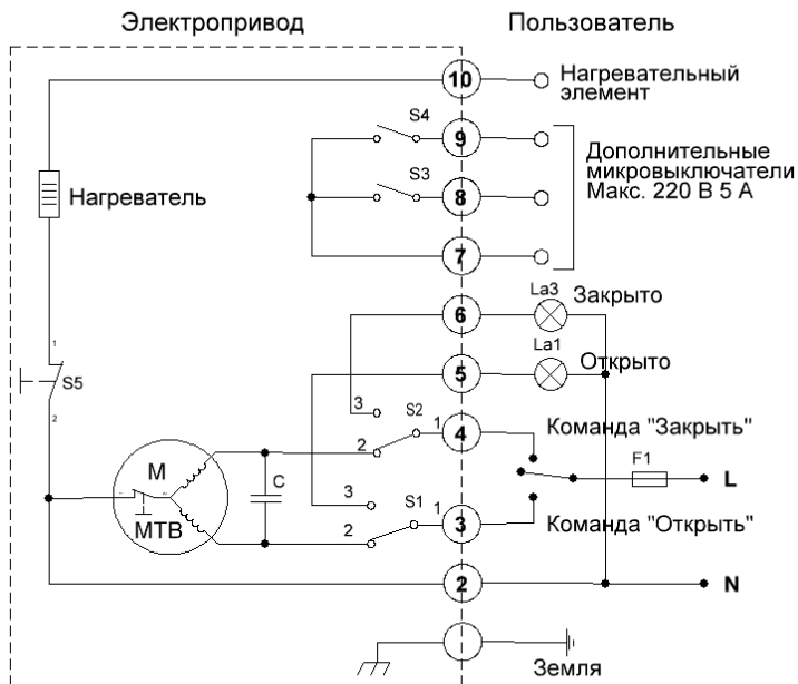
Рис. 2а Принципиальная электрическая схема подключения электропривода САТУРН ЭП-Ч(М) к сети 220 В, 50 Гц* (Исп. S1-стандартное, нагревательный элемент – опция, в ЭП-Ч 003 установка не возможна)
