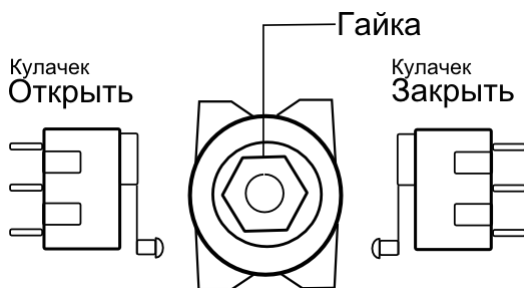
Рис. 86 Настройка концевых выключателей приводов САТУРН ЭП-Ч 020-100
