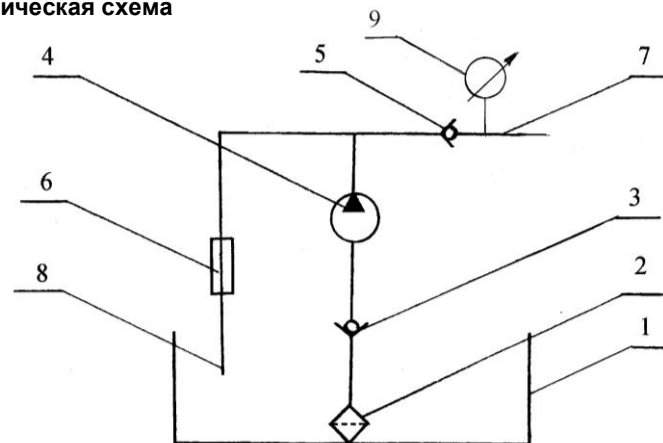
Гидравлическая схема
